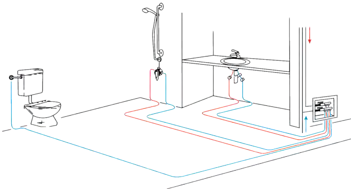
צנרת פקסליין עם אביזרי לחיצה לאספקת מים חמים וקרים בהתקנה שחילה
